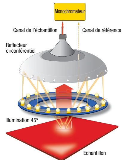
Principe de mesure du Datacolor 45G
